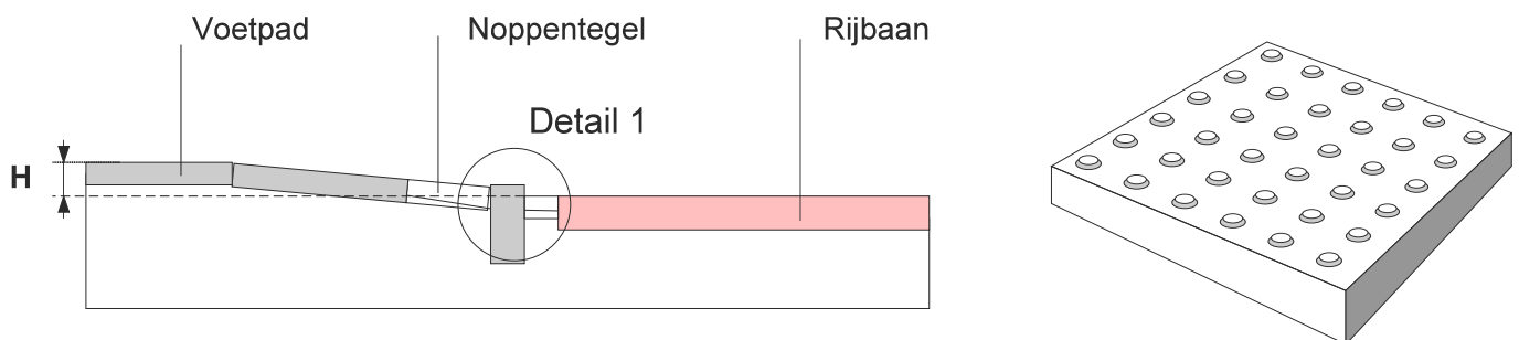
Doorsnede
